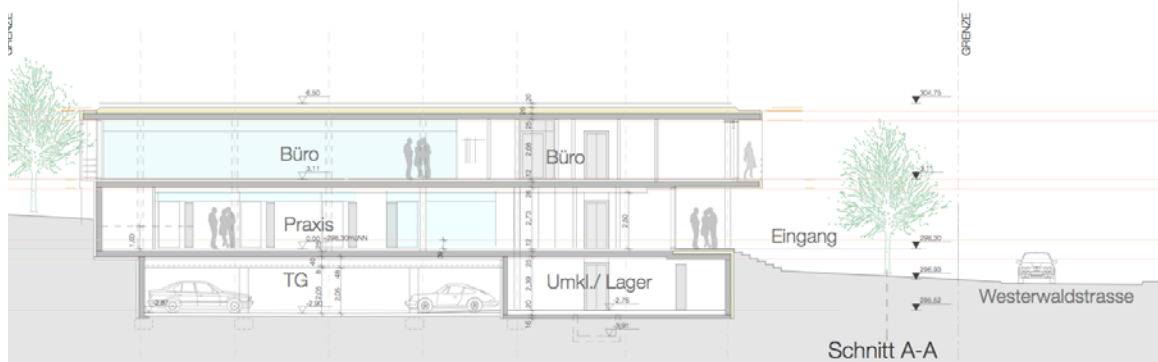
Vorhaben- u. Erschließungsplan, Schnitt, Ohlmeier Architekten BDA
